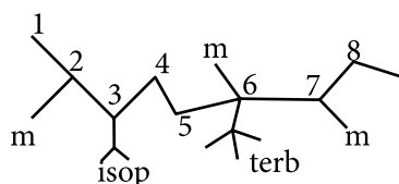
6-ter-butil-3-isopropil-2,6,7trimetilnonano
